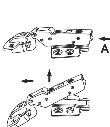
Схема демонтажа петли
